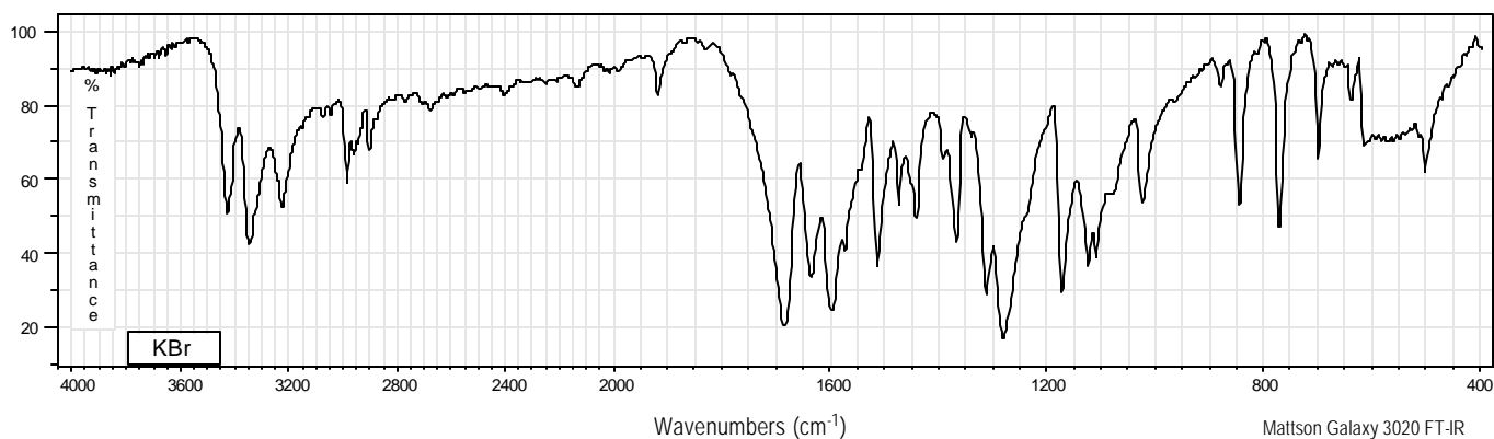
FT-IR
